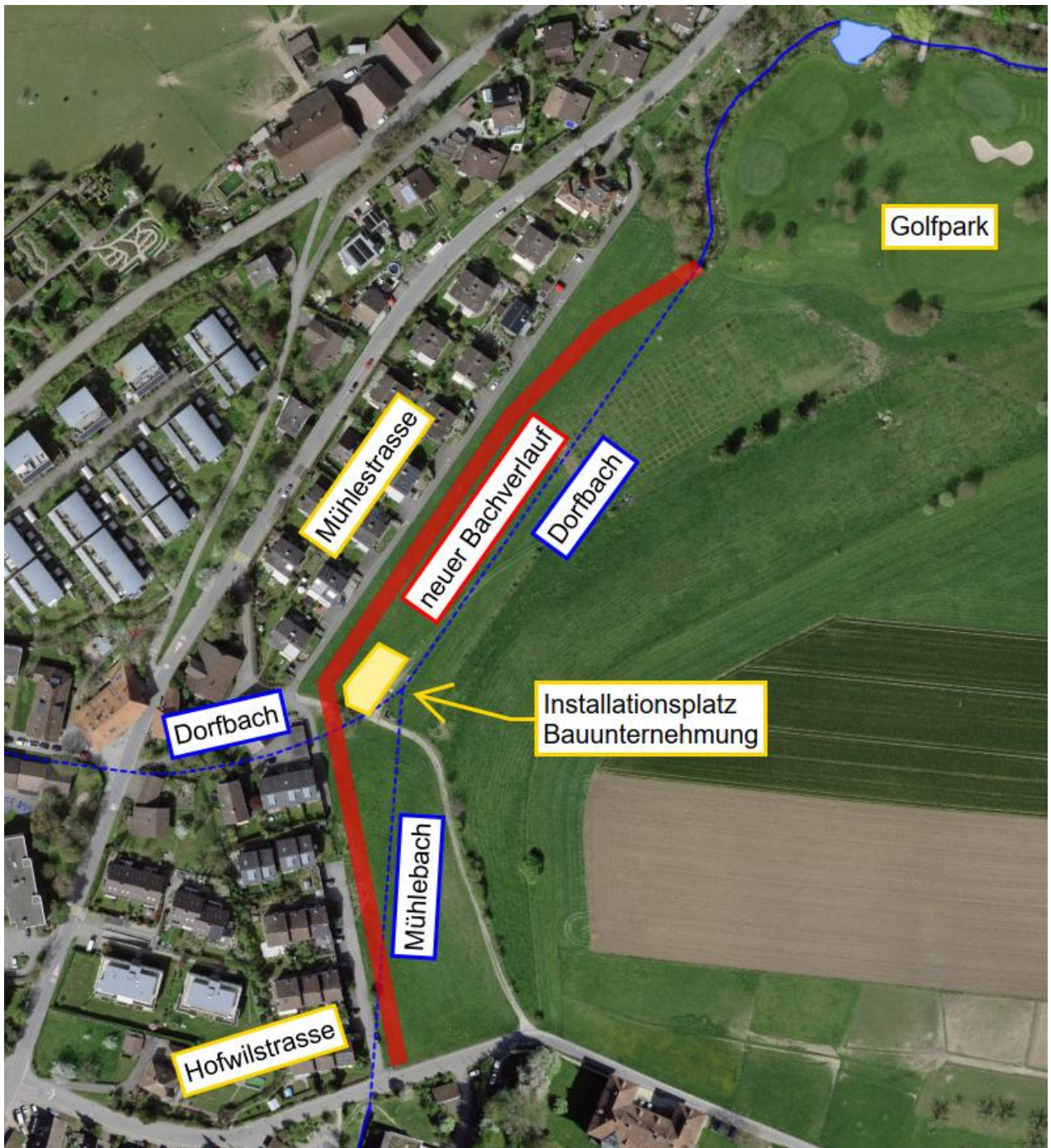
Abbildung 1: Übersichtsplan Revitalisierung Dorf- und Mühlebach
